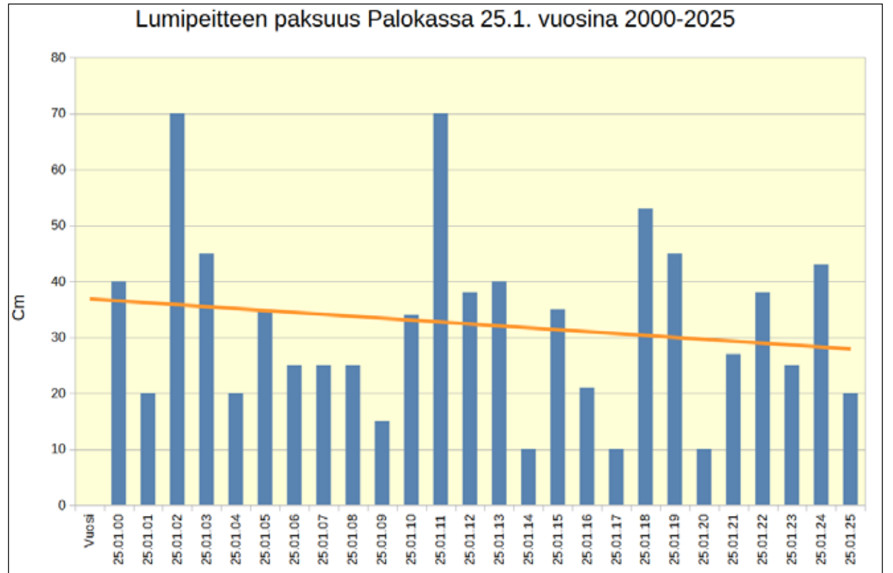
Diagrammiin on kuvattu lumipeitteen paksuus Palokan Terttumäessä vuosina 2000-2025. Havaintopäivä on 25.1.. Kuvassa on oranssin trendiviiva, joka kertoo lumikerroksen paksuuden muutoksesta havaintojakson aikana.
